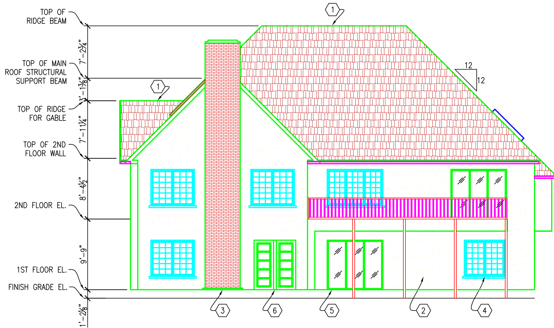
REAR ELEVATION SCALE: 1/8" = 1'-0"
