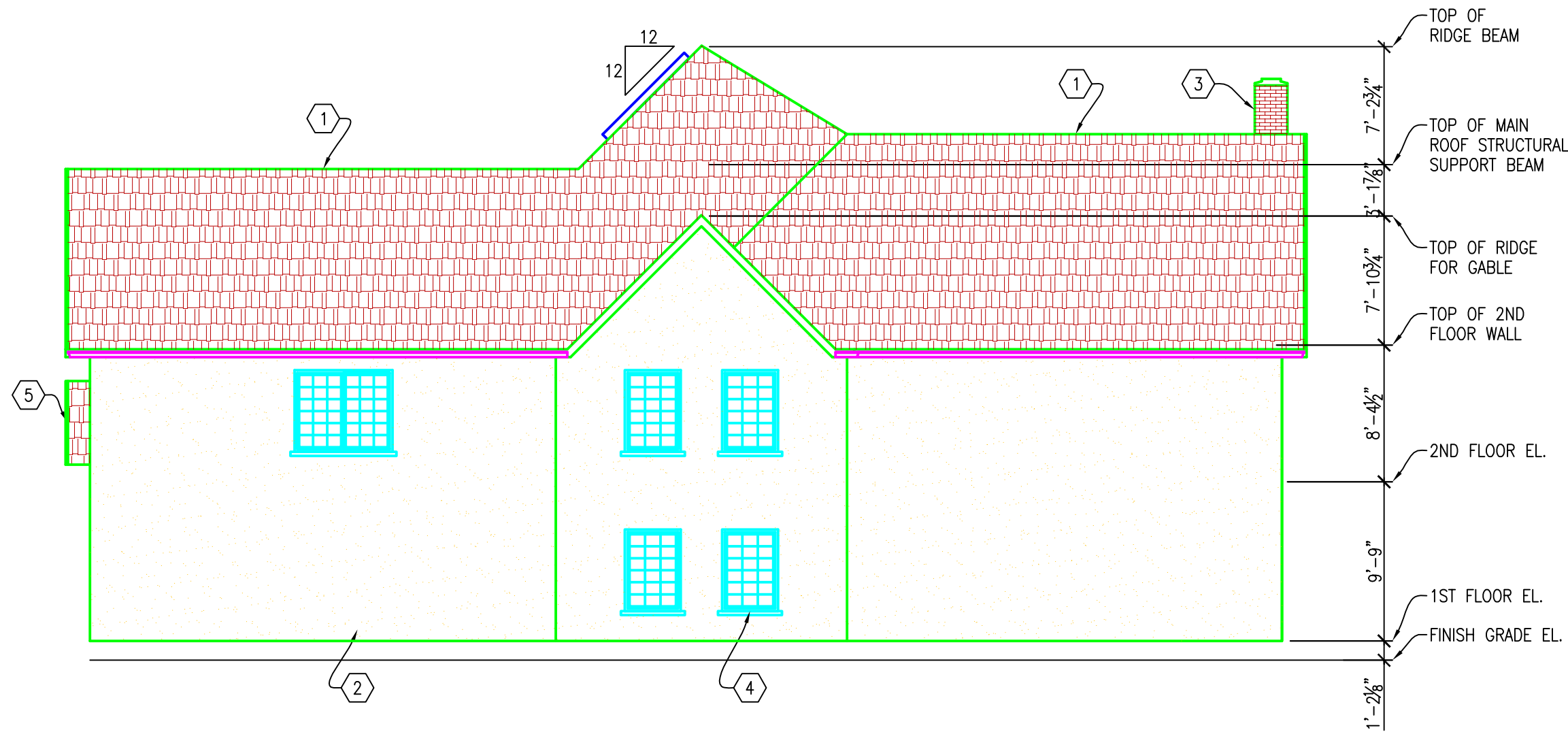
EAST ELEVATION SCALE: 1/8" = 1'-0"
