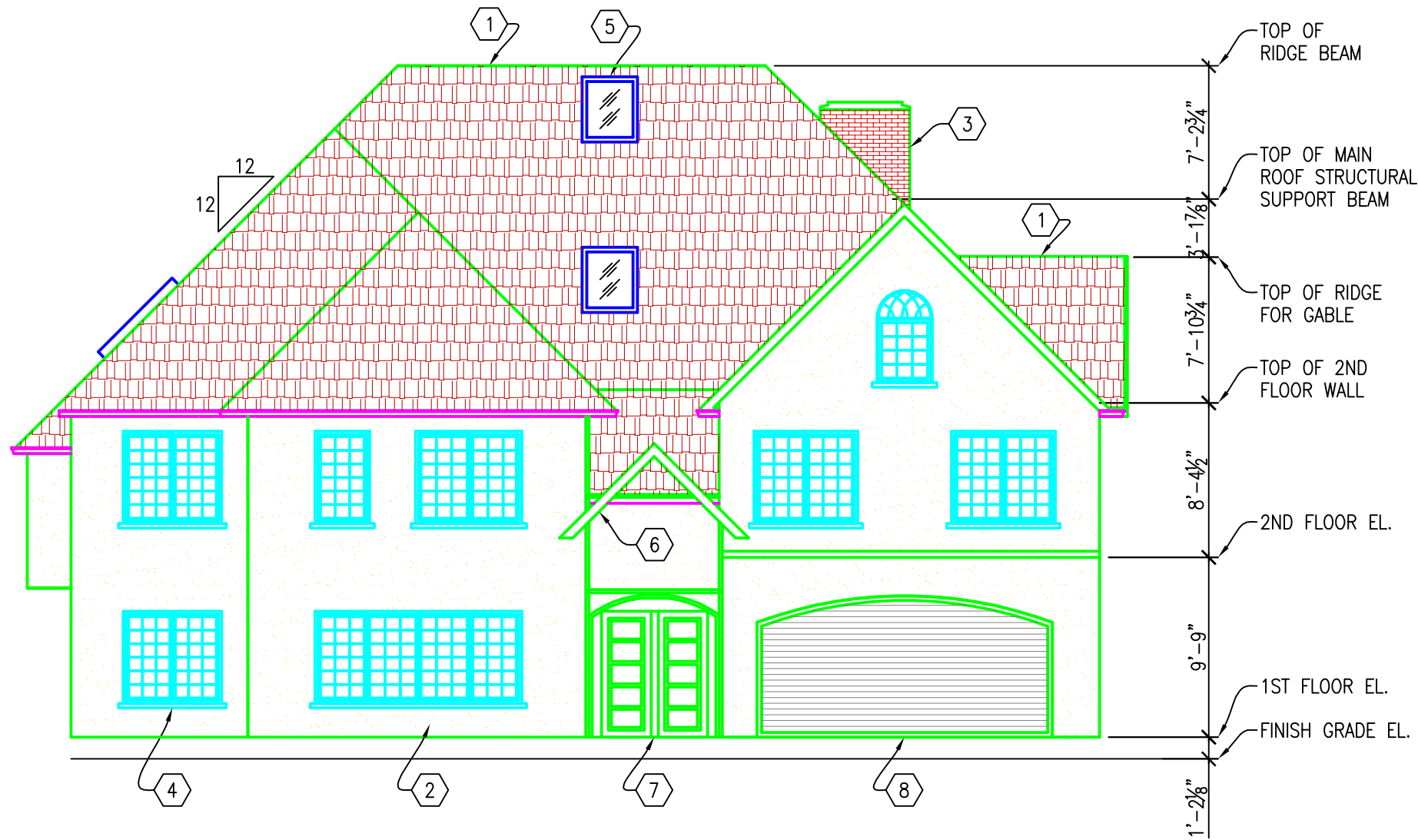
FRONT ELEVATION SCALE: 1/8" = 1'-0"
