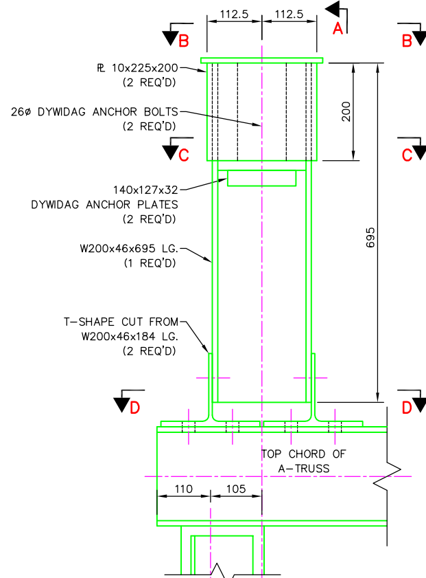
ELEVATION
