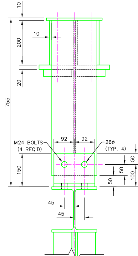
SECTION A-A
