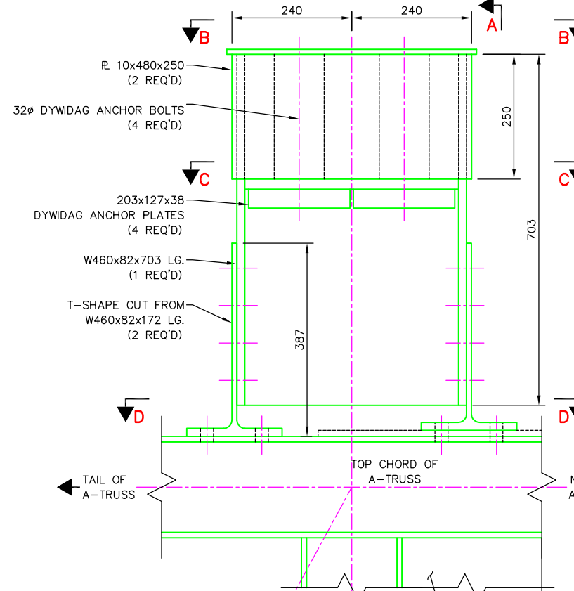
ELEVATION
