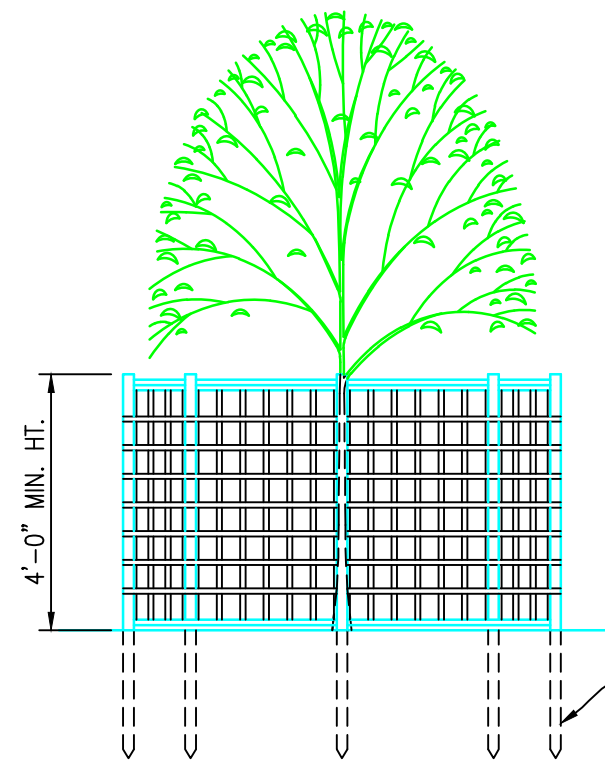
ELEVATION
